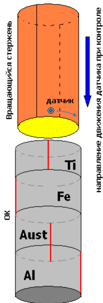
Образец №1 TP1. Схема расположения рисок в отверстии
