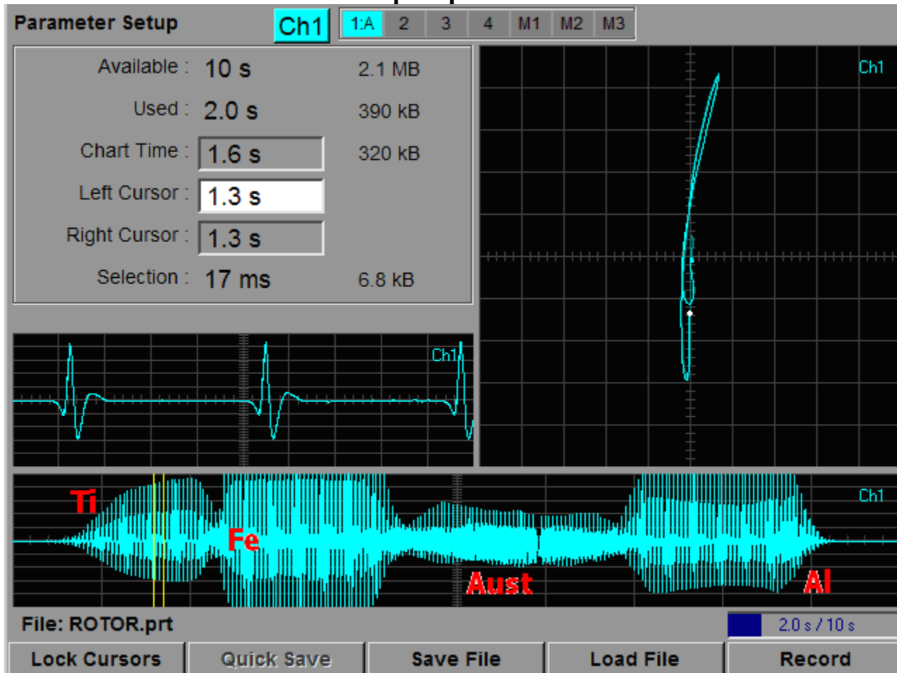
Рис. 3 Режим ленточной диаграммы с годографом.
