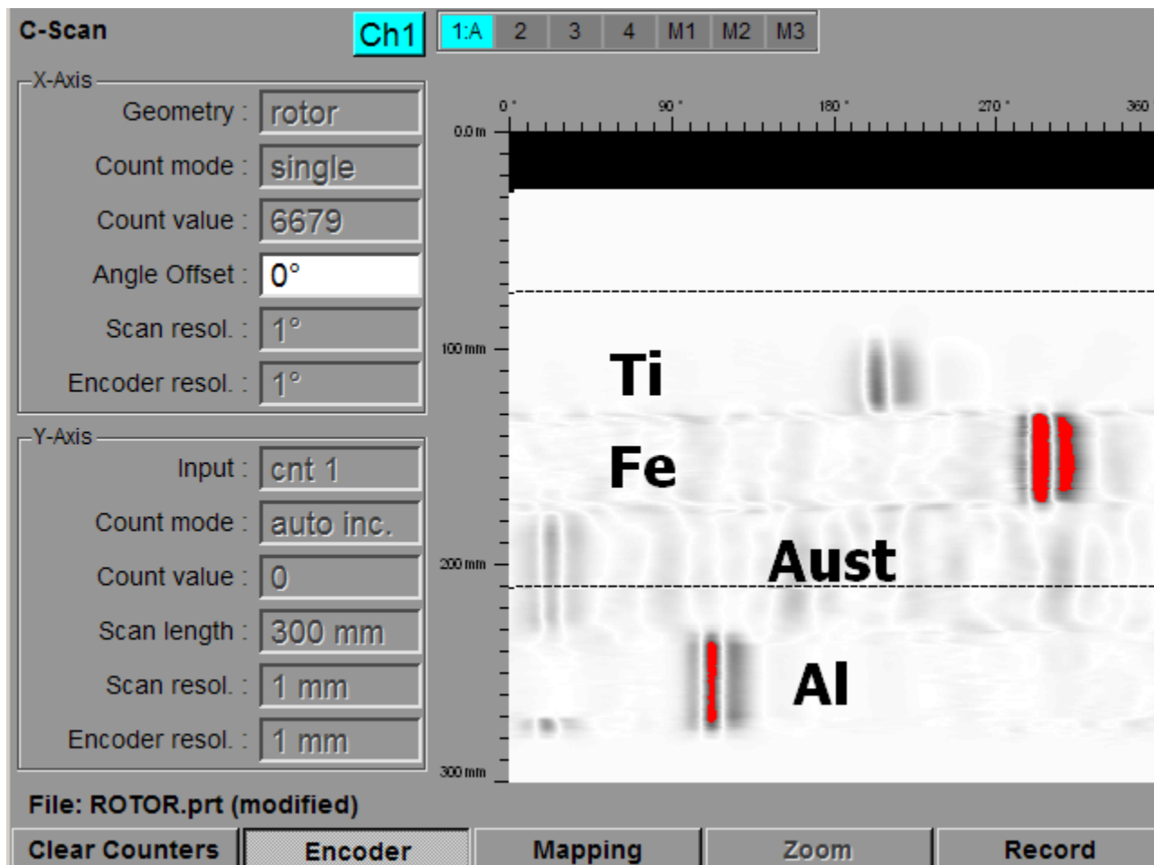
Режим С-скана
